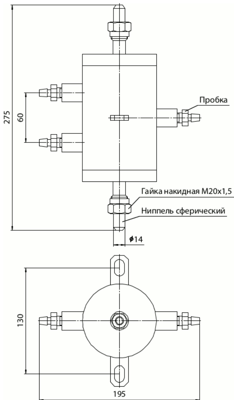
CP-25 Исполнение 4
