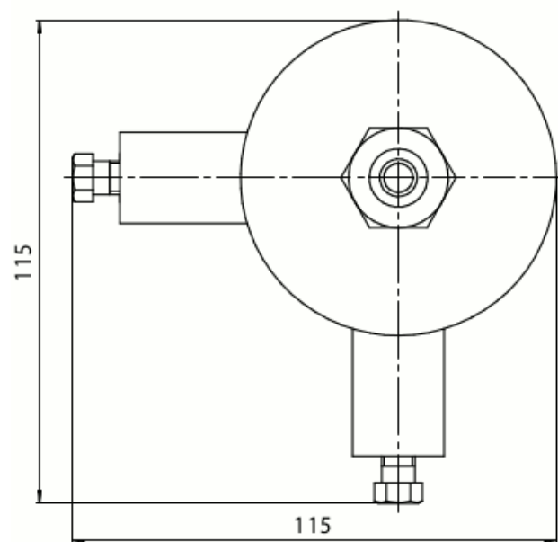
CP-25 Исполнение 2
