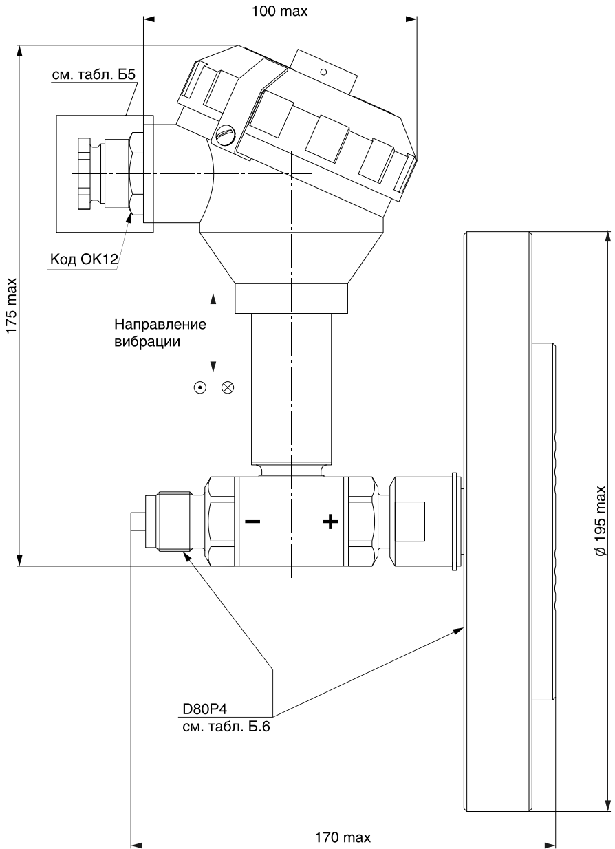
Рисунок Д.8 — Габаритные и присоединительные размеры датчика ЭНИ-12HS моделей ДГ
